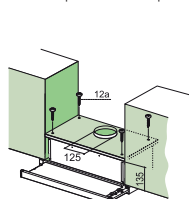
Montáž přes nosnou plochu
