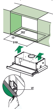
Montáž přes boční úchyty
