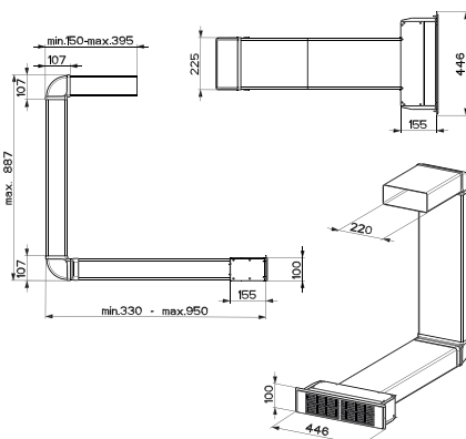
Sada pro recirkulaci přes mřížku 112.0539.570
