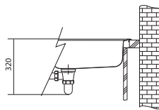
Přípravná deska BXX 210/110-45
